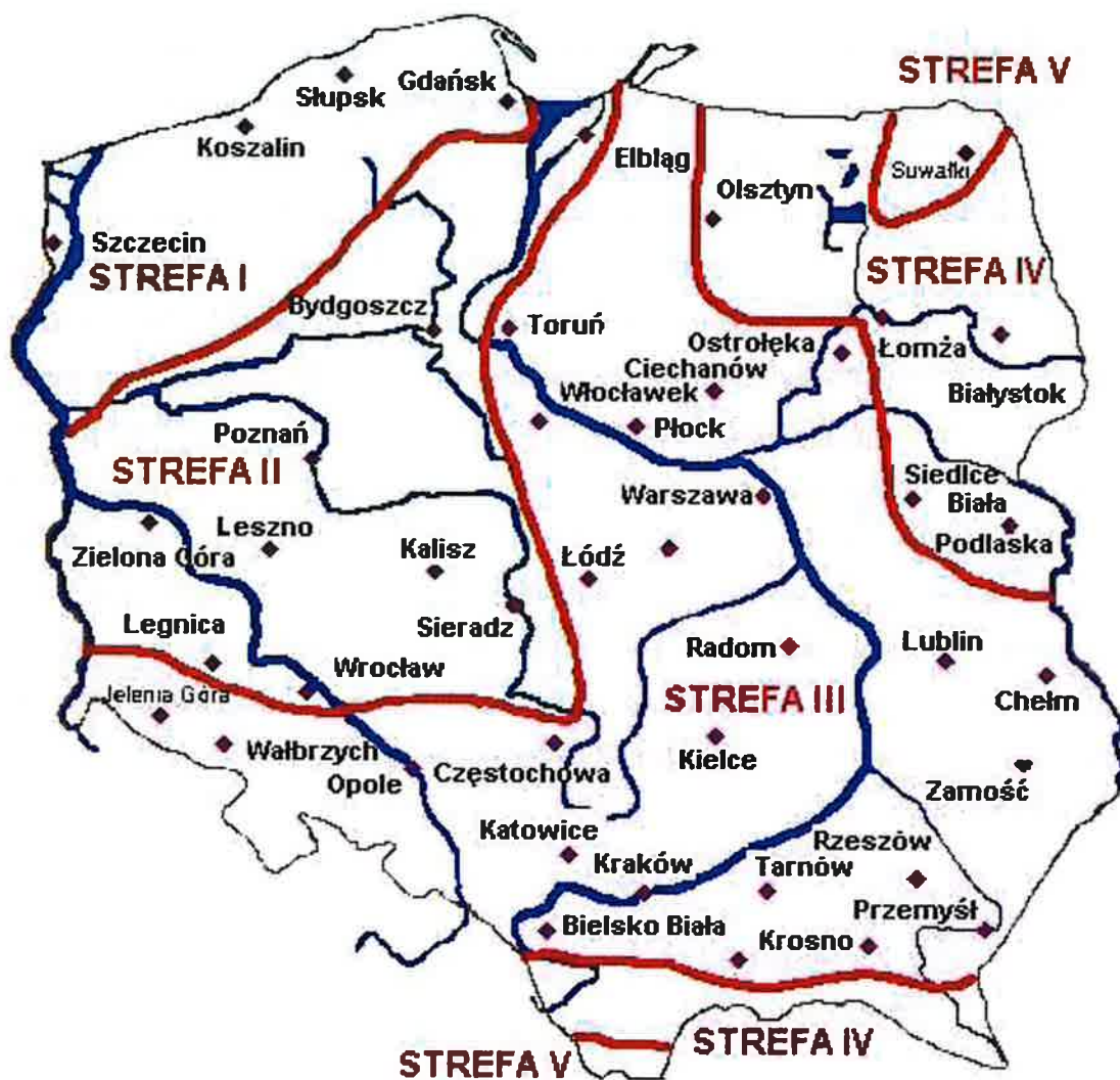
Rysunek 3 Strefy klimatyczne Polski
